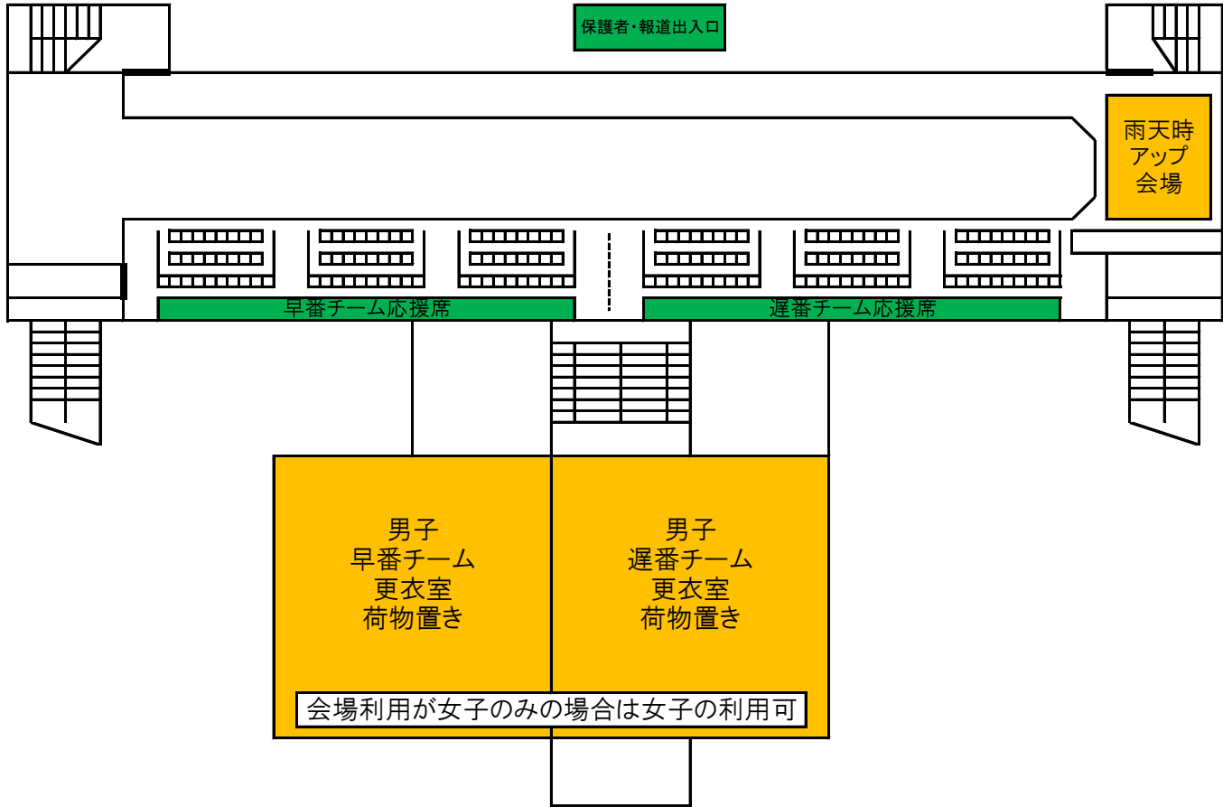
鹿央体育館 2階平面図
